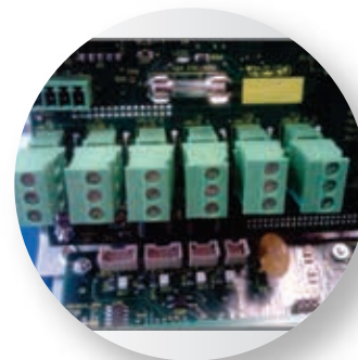
Conexión electroválvula
