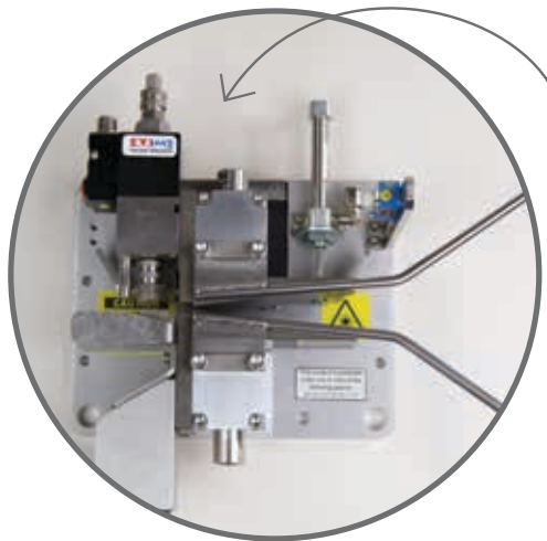
Válvula serie 900 en estación de encolado BoardRunner®
